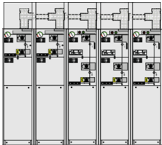
SafePlus ở dạng môđun toàn phần với hộp che thanh cái bên ngoài
