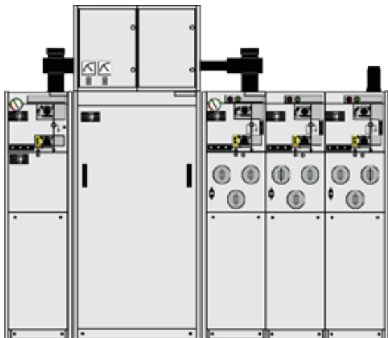
SafePlus với một lộ vào (môđun C), một môđun đo lường (môđun M) và ba nhánh chữ T có trang bị cầu chì (môđun Fs), sẵn sàng để mở rộng trong tương lai
