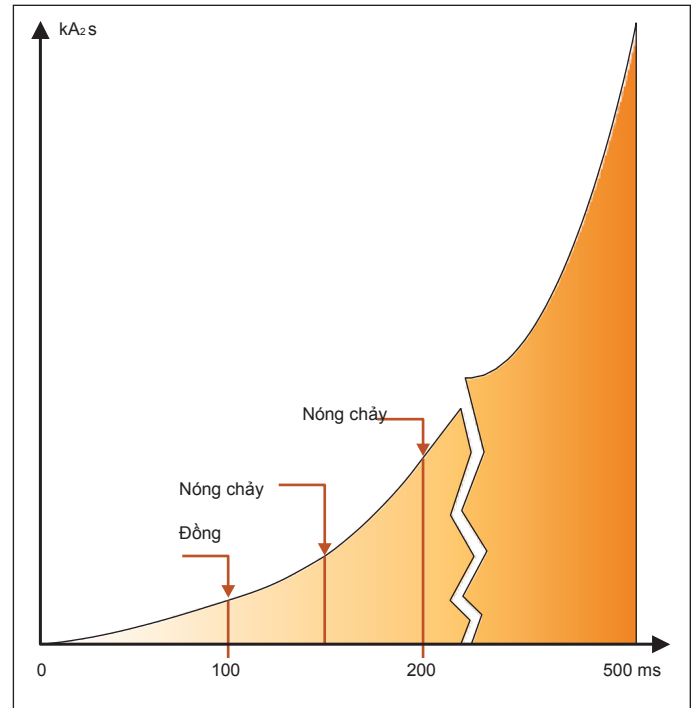
Khoảng thời gian hồ quang và hư hại gây ra
