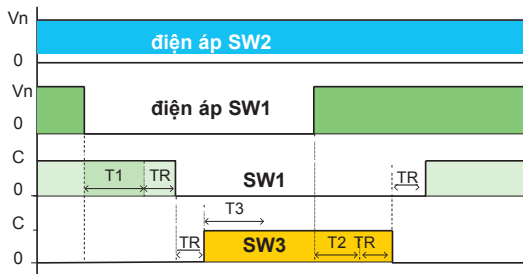
BTA - Chế độ tiêu chuẩn (không vận hành song song sau khi chuyển nguồn)
