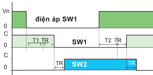
DM106851 ATS nguồn Lưới: Chế độ tự động (vận hành song song sau khi tự động chuyển nguồn)
