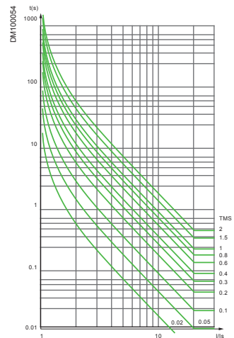
Đường thời gian cực dốc của IEC (IEC/EIT hoặc IEC/C)
