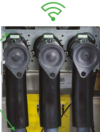
Các cảm biến TH110 lắp trên các điểm nối cáp
