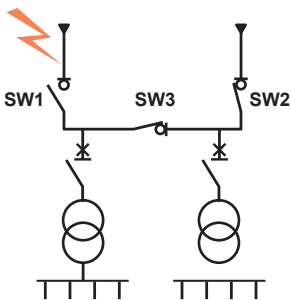
BTA - Chế độ tiêu chuẩn (không vận hành song song sau khi chuyển nguồn)
